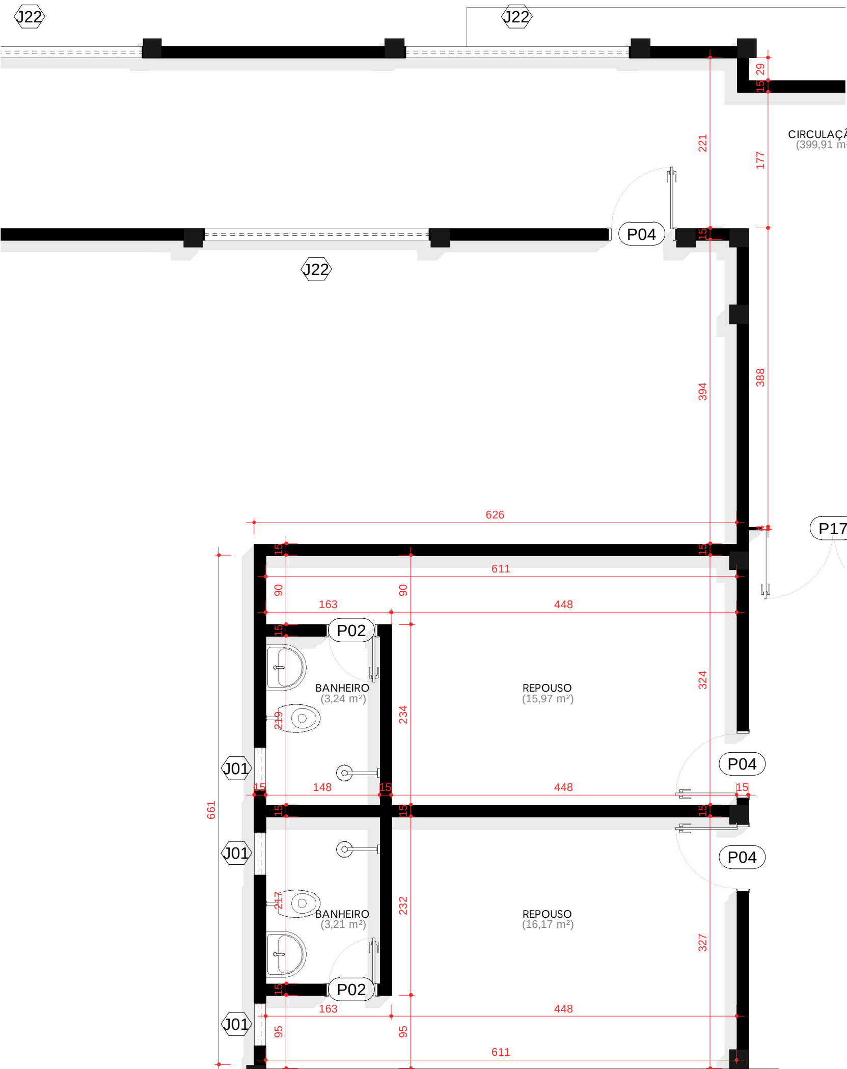
PLANTA BAIXA DETALHES - BLOCO 02/1 ESC: 1 : 50
