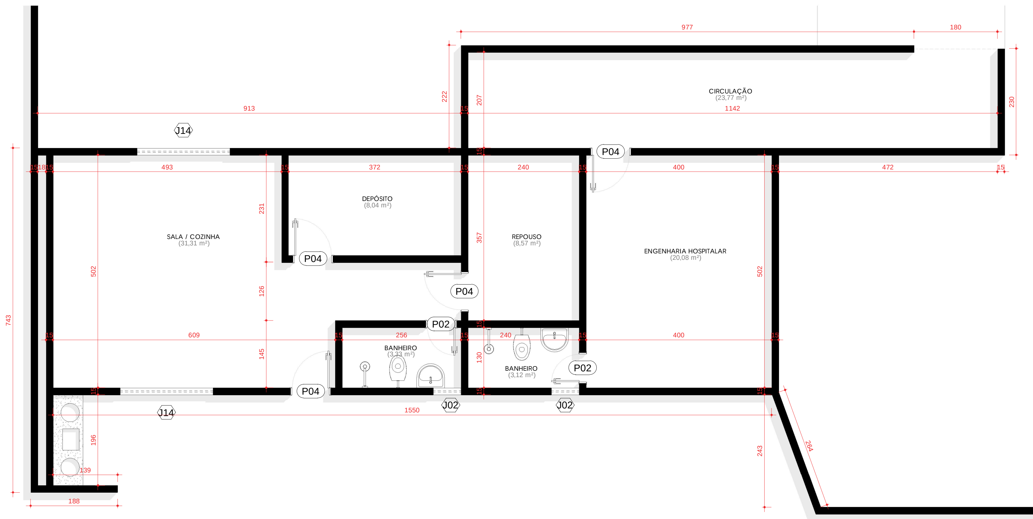
PLANTA BAIXA DETALHES - BLOCO 05/2 ESC: 1 : 50
