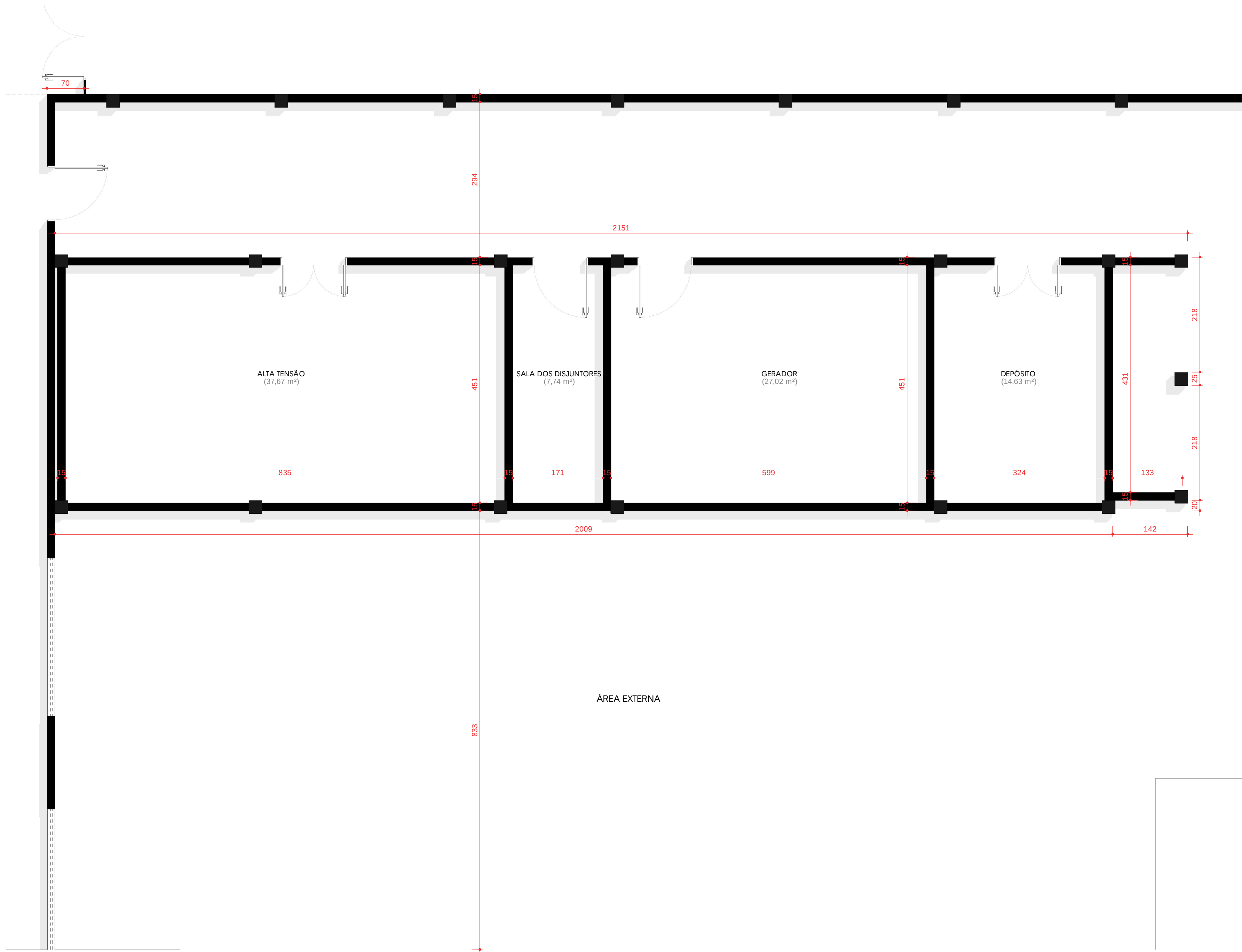
PLANTA BAIXA DETALHES - BLOCO 03/2 ESC: 1 : 50
